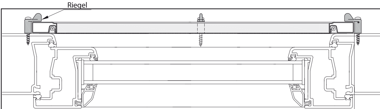
Horizontaler Schnitt
