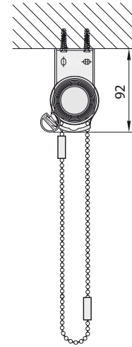
Detail Deckenmontage
